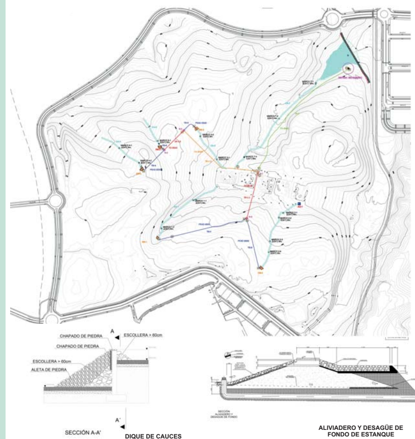
CIRCUITO DE CAUCES ORNAMENTALES
