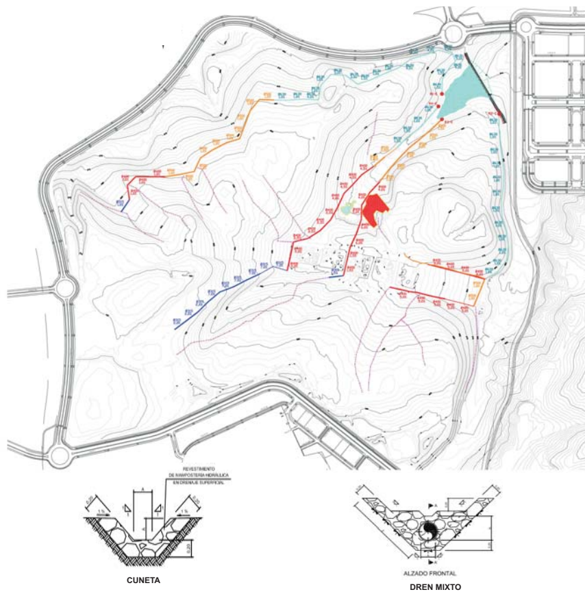
RED DE SANEAMIENTO
